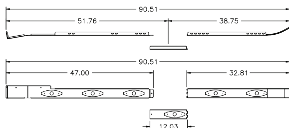
EMPLACEMENT DE LA TRAPPE À CARBURANT - CÔTÉ PASSAGER
